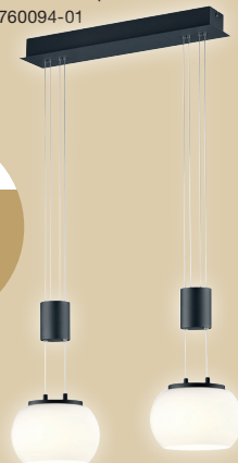
LED-Jojo-Pendelleuchte, 2-flg., B./H. ca. 52/150 cm, Alu schwarz/Glas weiß, Switch-Dimmer, höhenverstellbar, 2x8W LED (2x800 Lumen) 3000K. 69760094-01
